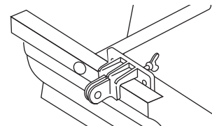
Przymocuj wspornik do rynny lub muru
