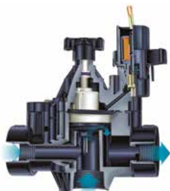
Przekrój zaworu PGA
