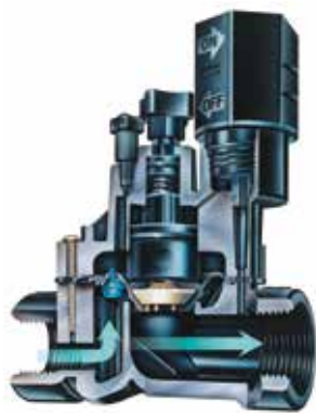
Przekrój elektrozaworu DVF
